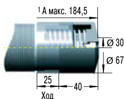
Защитный колпачок
