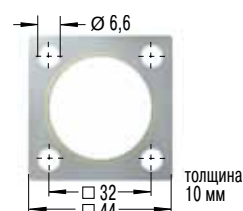
Квадратный фланец
