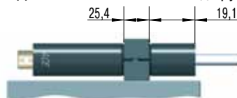
Перегородочное крепление для VC25...F с крепежным блоком KB... (доступен корпус 23,8 мм без резьбы)
