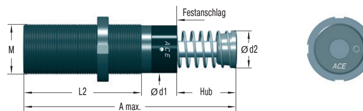
Gewinde UNF 1 3/4-12 (Bestellbezeichnung ohne Endung -M)
